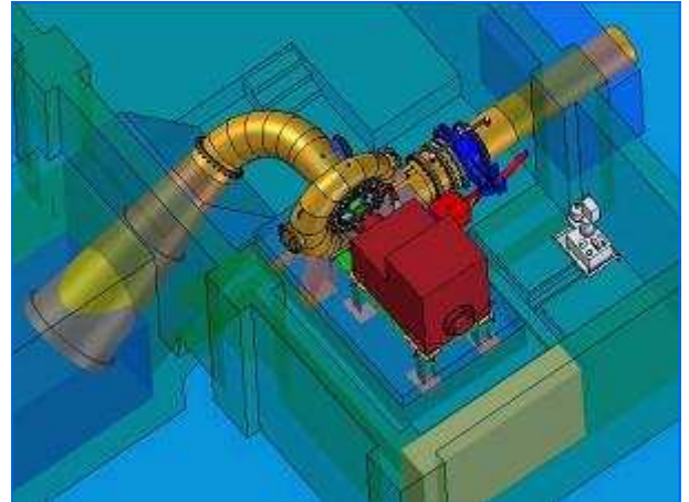
CAD Einbauskitze CAD Installation draft
