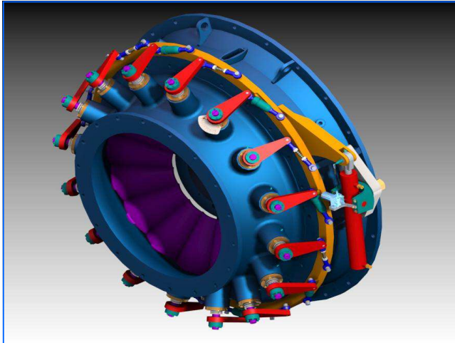
Leitapparat 3D guide vane apparatus 3D
